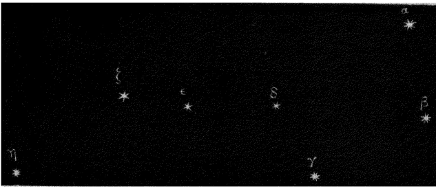
FIG. 17. URSA MAJOR.
