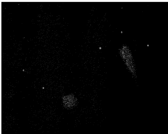
FIG. 26. 75 H. II. VIRGINIS.
