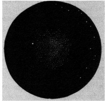
FIG. 43. 56 M. LYRÆ.
