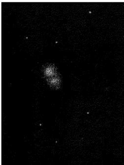
FIG. 14. 57 \mathbb{H} . I. LEONIS.
