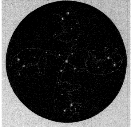
FIG. 30. URSA MINOR.
