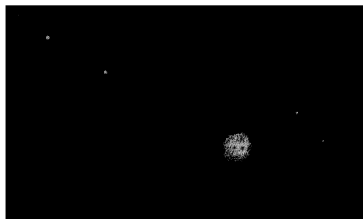
FIG. 7. 26 \mu . IV. ERIDANI.
