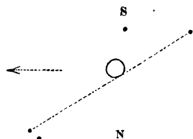
FIG. 16. 27 H. IV. HYDRÆ.
