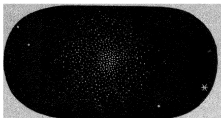
FIG. 34. 13 M. HERCULIS.
