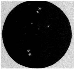
FIG. 40. \epsilon LYRÆ.
