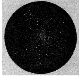
FIG. 31. 5 M. LIBRÆ.
