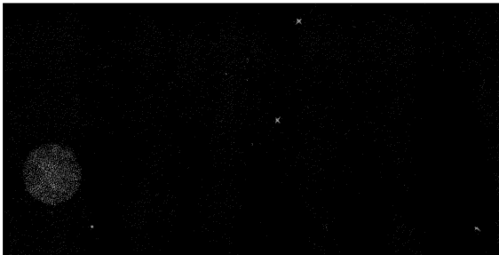
FIG. 18. 97 M. URSÆ MAJORIS.
