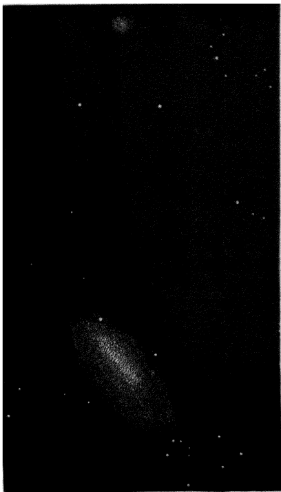
FIG. 1. 31 M. ANDROMEDÆ.
