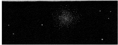
FIG. 46. 15 M. PEGASI.
