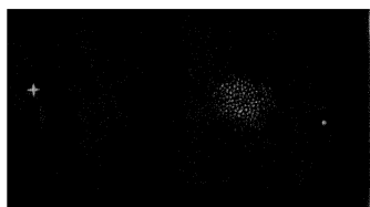
FIG. 36. 92 M. HERCULIS.
