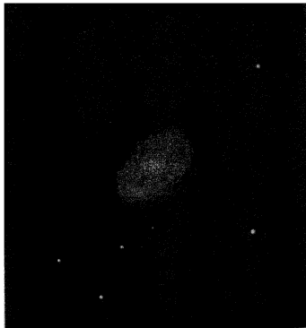
FIG. 8. 1 M. TAURI.
