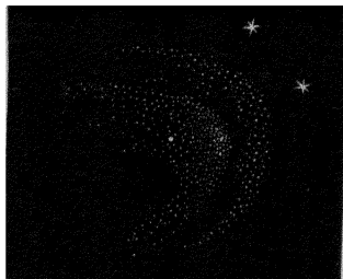
FIG. 41. 11 M. ANTINOI.
