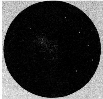
FIG. 13. 67 M. CANCRI.
