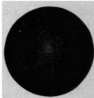
FIG. 48. 30 M. CAPRICORNI.
