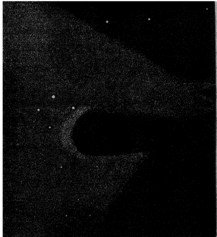
FIG. 9. \theta^1 ORIONIS.
