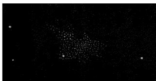
FIG. 49. 52 M. CEPHEI.
