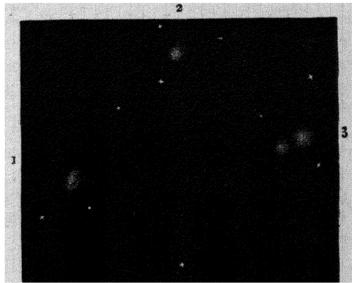
FIG. 25. 60 M. VIRGINIS. 4
