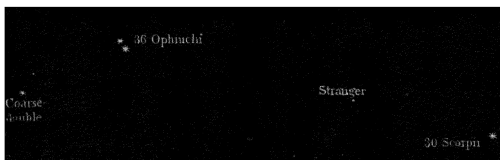
FIG. 35. 36 OPHIUCHI.
