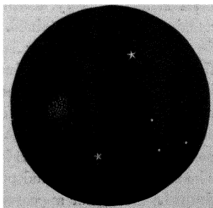
FIG. 32. 80 M. SCORPII.
