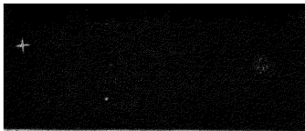
FIG. 38. 37 \mu . IV. DRACONIS.
