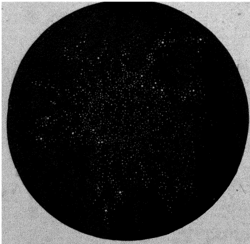
FIG. 50. 30 H VI. CASSIOPEIÆ.
